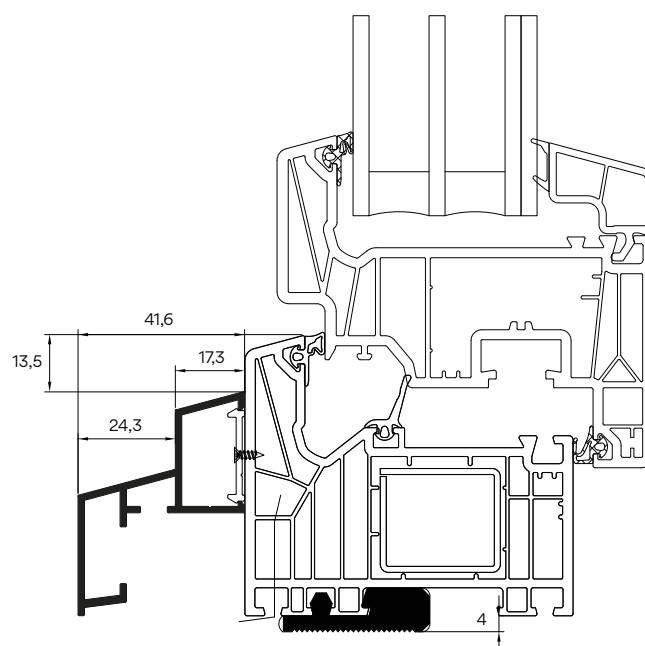
Dorpel AD01-S (epdm)*
