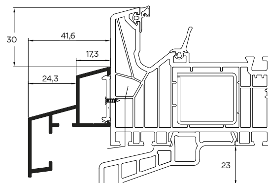
Dorpel AD01-S (9295/23)
