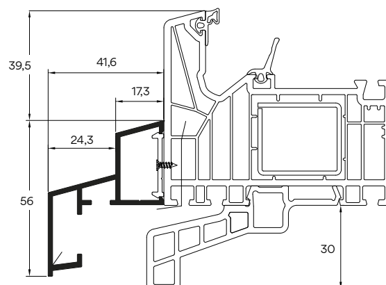
Dorpel AD01-S (9295/30)
