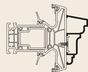
Tussenregel AD06T
