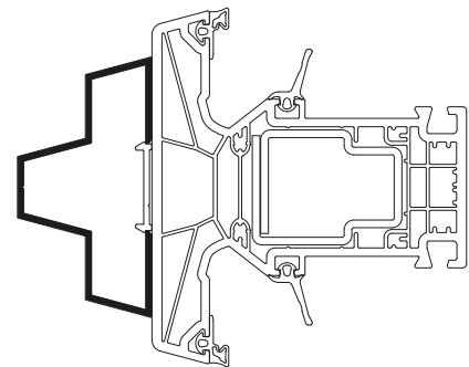
Tussenregel AD06-S
