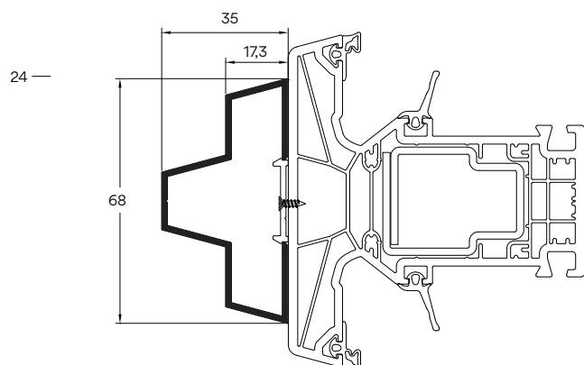
Tussenregel AD06-S
