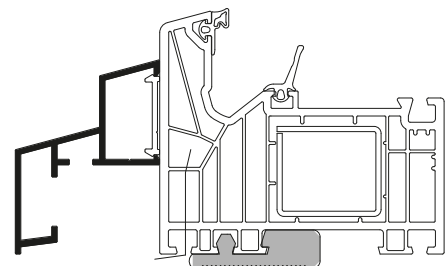
Dorpel AD01-S
