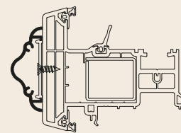
Makelaar AD03M2
