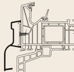
Dorpel AD05K1
