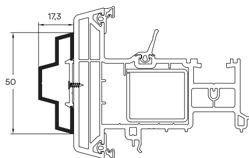
Makelaar AD03-S
